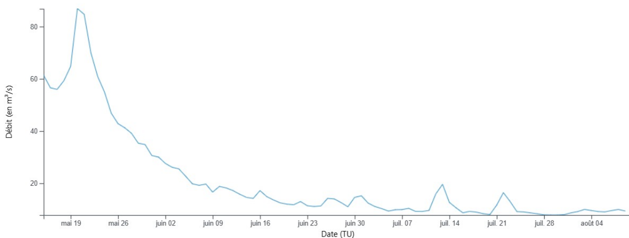
Figure 5: Courbe des débits de l'Allier au niveau de Vieille-Brioude en fonction de la date sur la période de l'étude (Source: HydroPortail)
